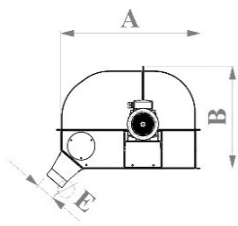
Üst Başlık-Upper Head of Elevator-Верхний башмак
